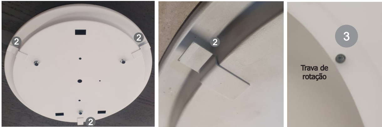
Imagem ilustrativa - Difusor Versão G
