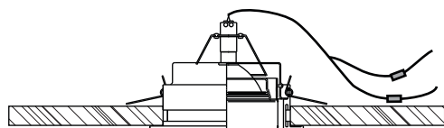
Luminária instalada.
